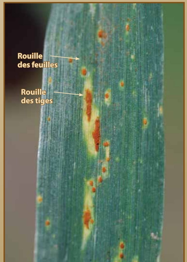
Figure 2. Comparaison des lésions de la rouille des tiges et de la rouille des feuilles sur les tissus foliaires. Notons la plus grande superficie en forme de diamant de la rouille de la tige par rapport à la rouille des feuilles.
