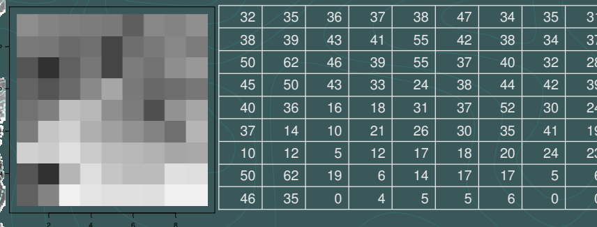
Data Values
